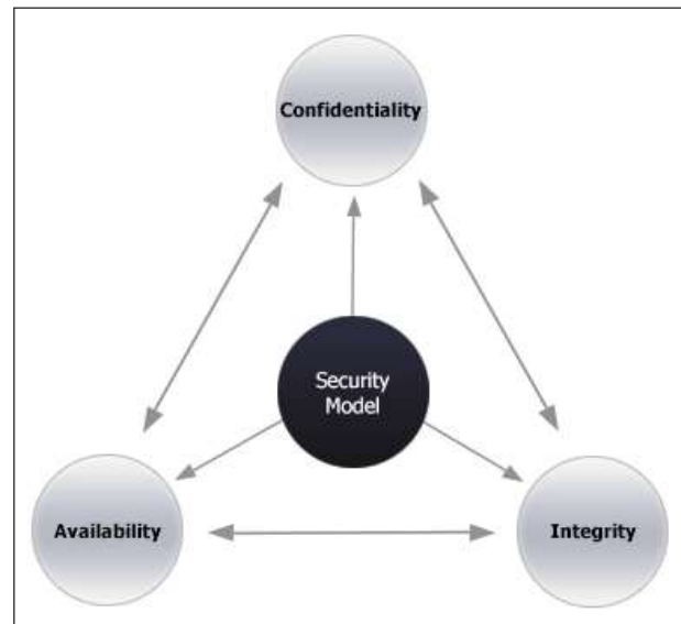
Fig. 1: CIA Triad
